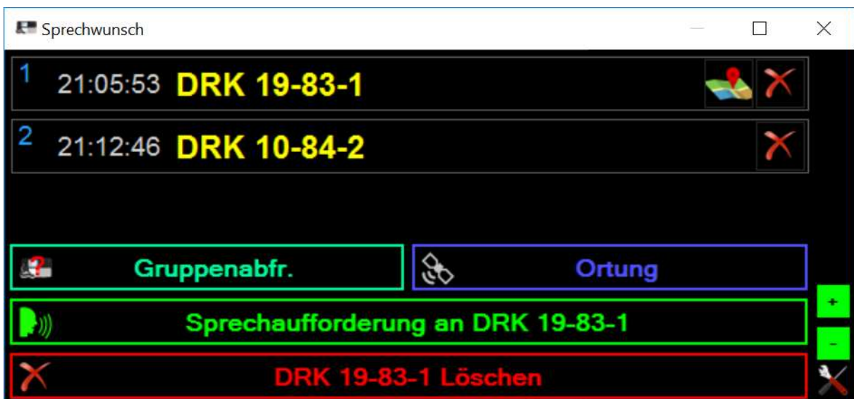
Abbildung 14 - Sprechwunschanzeige
