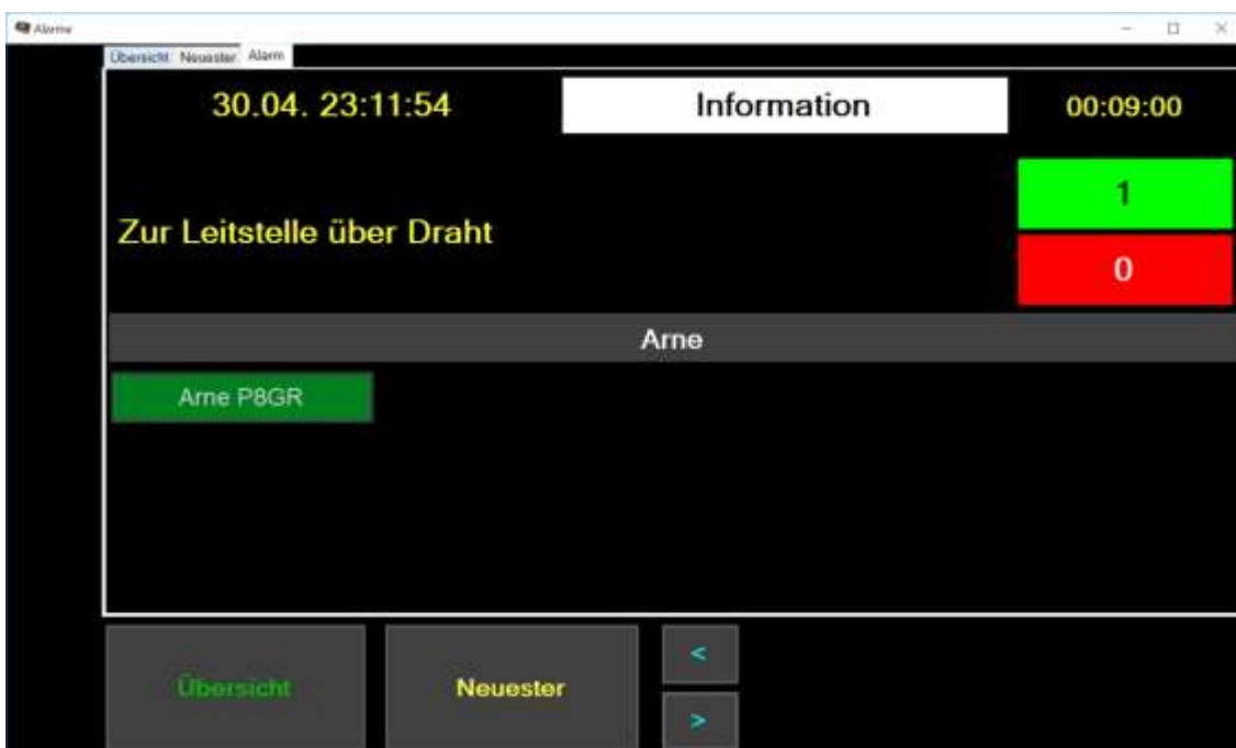
Abbildung 11 - Alarm Detailanzeige
